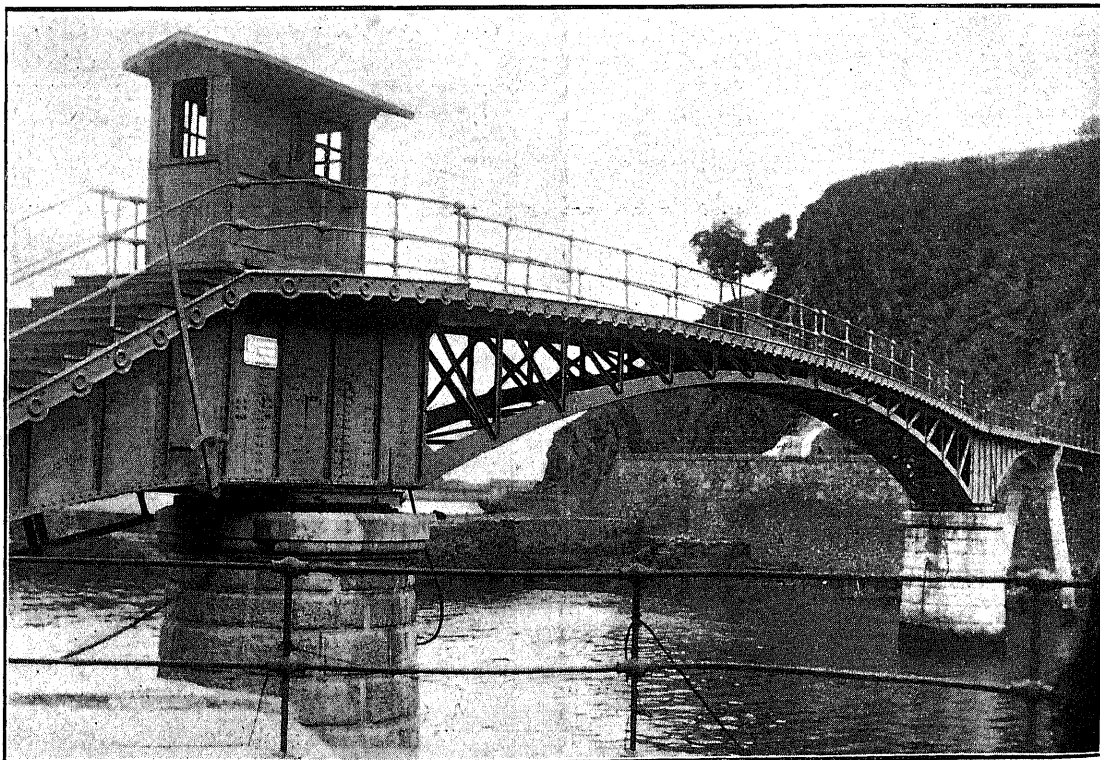
ONDARROA — (Bizkaya). Nuevo puente giratorio recientemente inaugurado.
