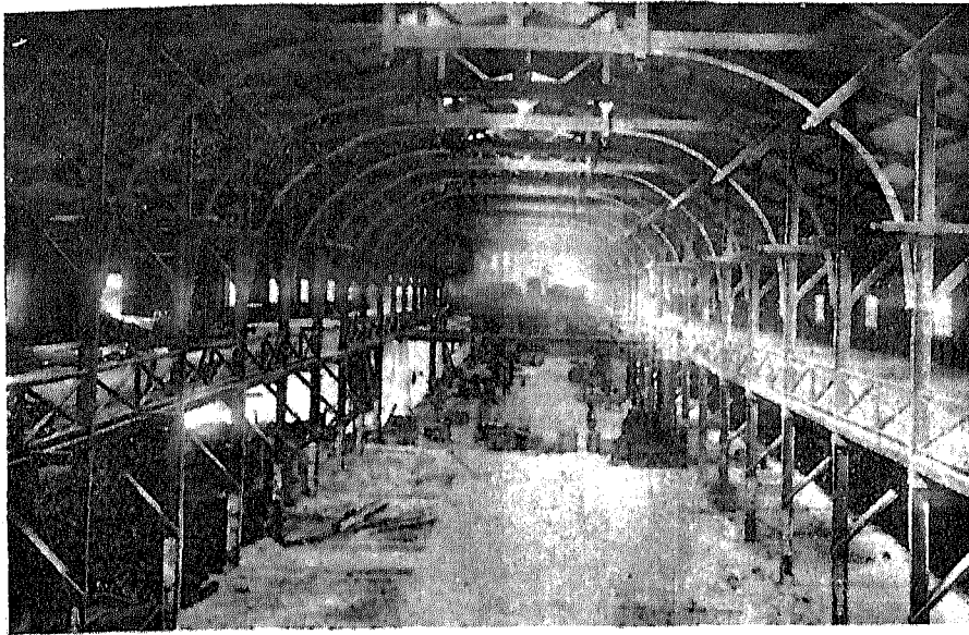
El cobertizo de los talleres de Barracas.—Preparando los cimientos para las máquinas
