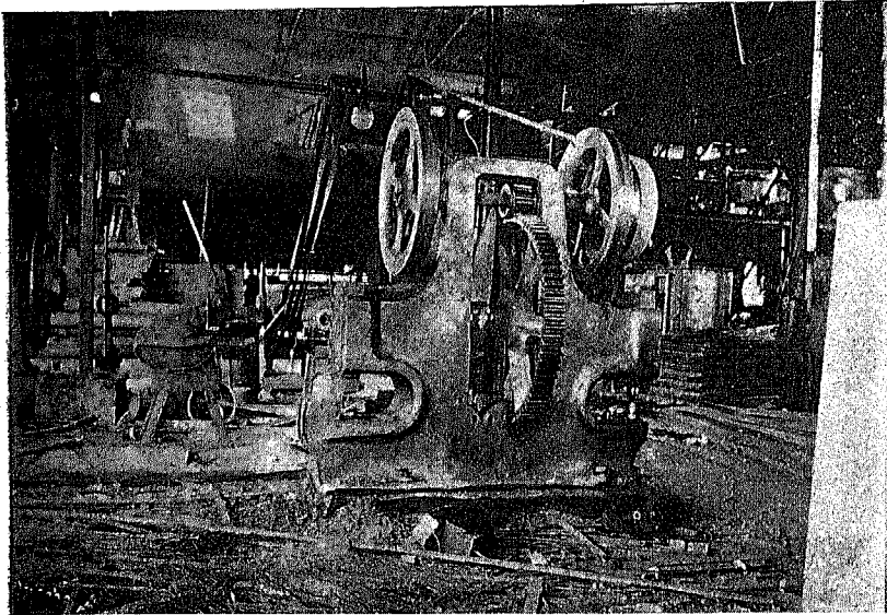
Máquina para cortar ángulos y planchernas.—Talleres del Paseo de Julio
