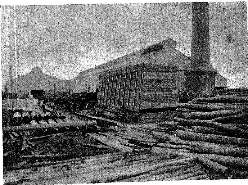
Fondo de los Talleres y Enfriador.—(Barracas al Sur)
