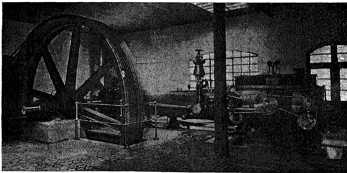
Mótor de los talleres de Barracas al Sur
