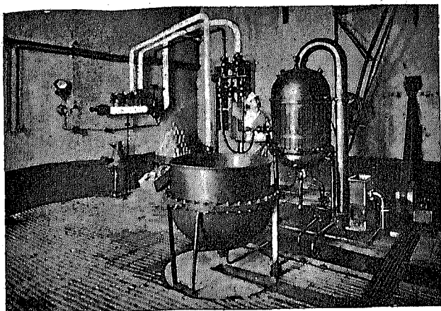
Fabricación de leche condensada y dulce de leche
