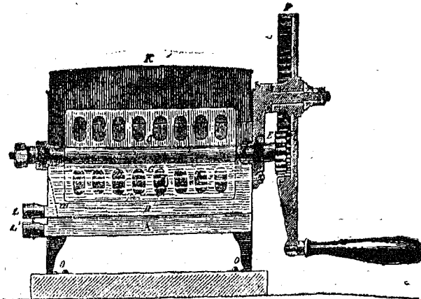
Fig. 8.—Mantequera Girad
