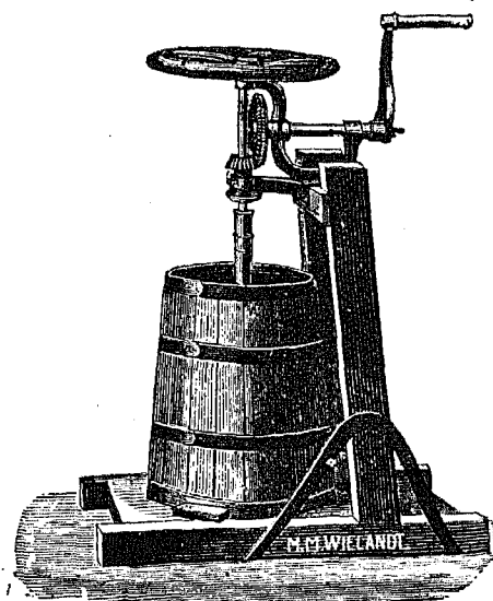
Fig. 6.—Mantequera
