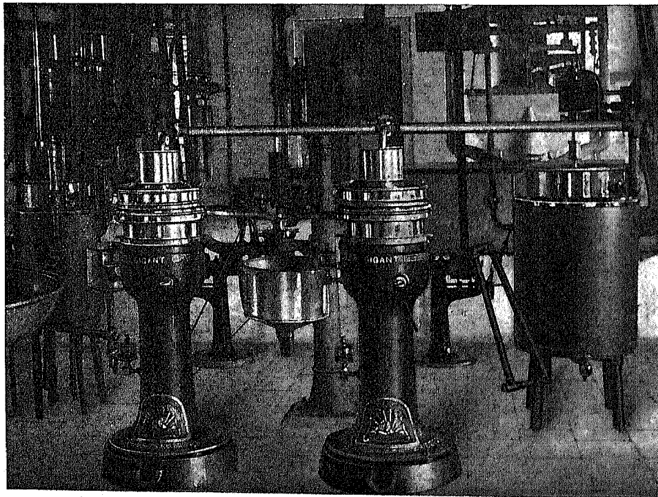
INDUSTRIA LECHERA—Saln de desnatadoras
