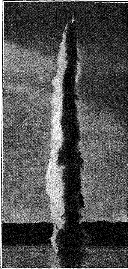
Explosión de una mina sub-marina de 100 libras de algodón pólvora y 100 de dinamita
